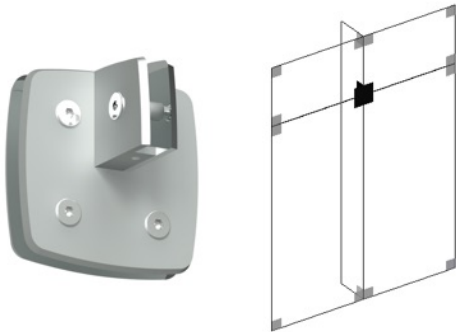
1319 Cantoneira Quádrupla em Angulo
