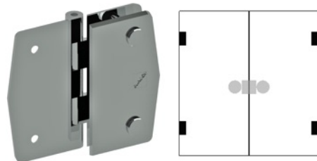
3146 Dobradiça Porta Modelada com Aba Reta
