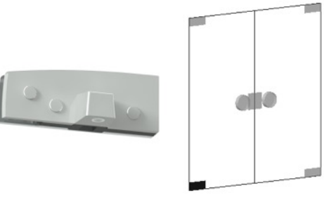
1109 Dobradiça Inferior Excêntrica Esquerda
