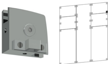
1525 Contra Trinco para 1513
