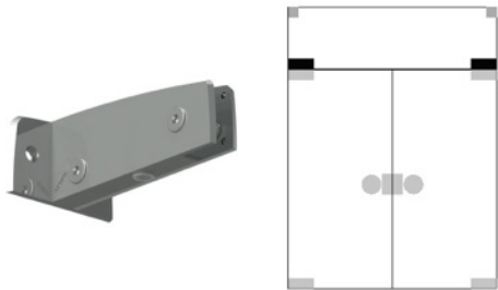
1207 Suporte Excêntrico Esquerdo
