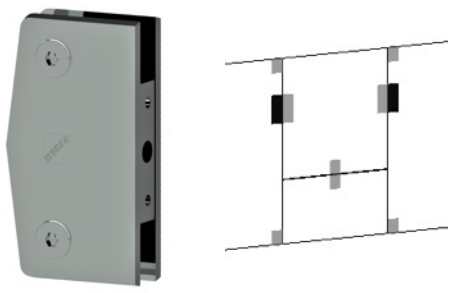
3421 Suporte para Dobradiça Pivotante (Pequena)
