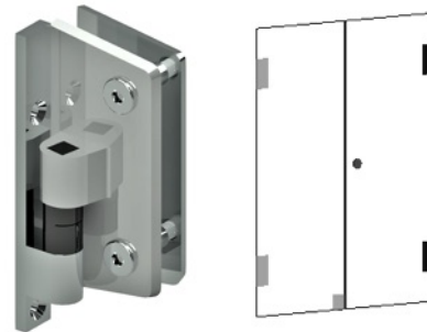
3714 Dobradiça Automática Direita Pq (1 furo)
