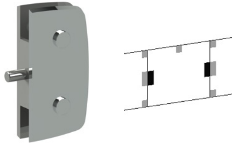
1136 Dobradiça Lateral Excêntrica (Pequena)
