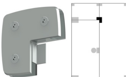
1315 Suporte Triplo com Aparador
