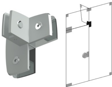
1311B Suporte Triplo Contravento Simples Desl. Dir.
