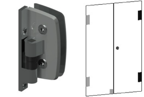
1115D Dobradiça Dupla Vidro/Vidro Direita
