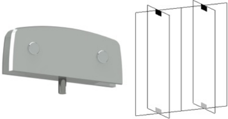
1113 Dobradiça Pivotante Inferior com Trinco
