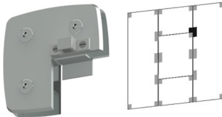
1311 Suporte Triplo Contravento Simples Direito
