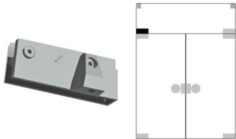
3129 Suporte L em Ângulo Esquerdo
