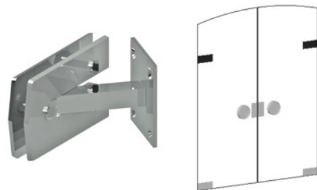
3146 Dobradiça Porta Modelada com Aba Reta
