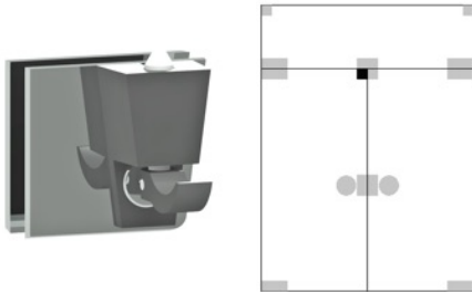
3250 Mini Trinco para Janela
