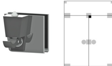
3251 Espelho para Trinco (para 3250)
