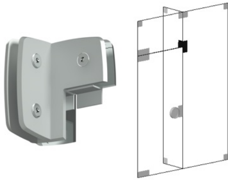
1314A Suporte Triplo Contravento Duplo Esq c/ Ap.
