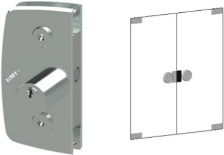
1520 TETRA Fechadura Central Tetra
